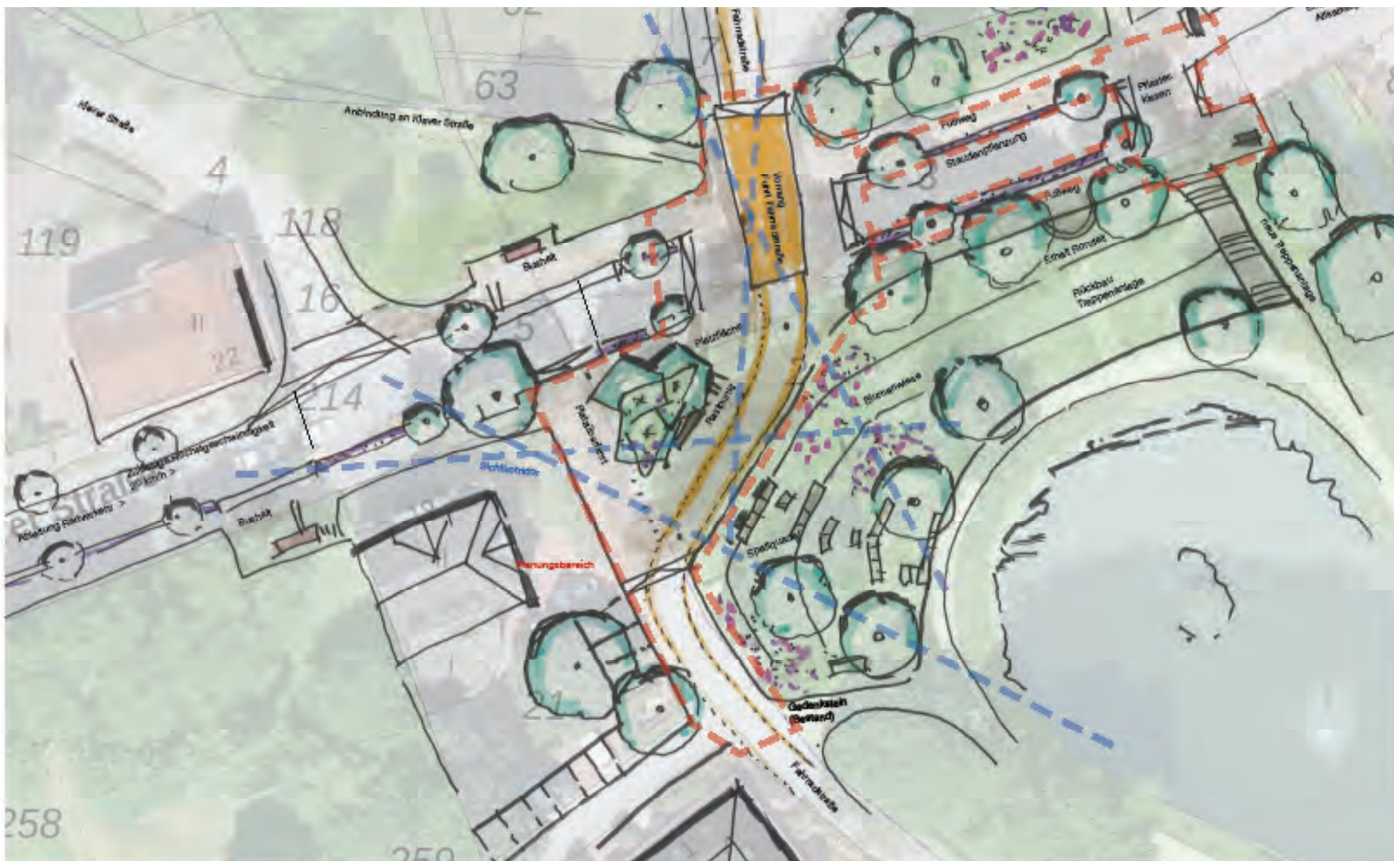
Wallanlagen Kalkar Post II 06 | Juni 2023 | Planungsbüro DTP Landschaftsarchitekten GmbH
