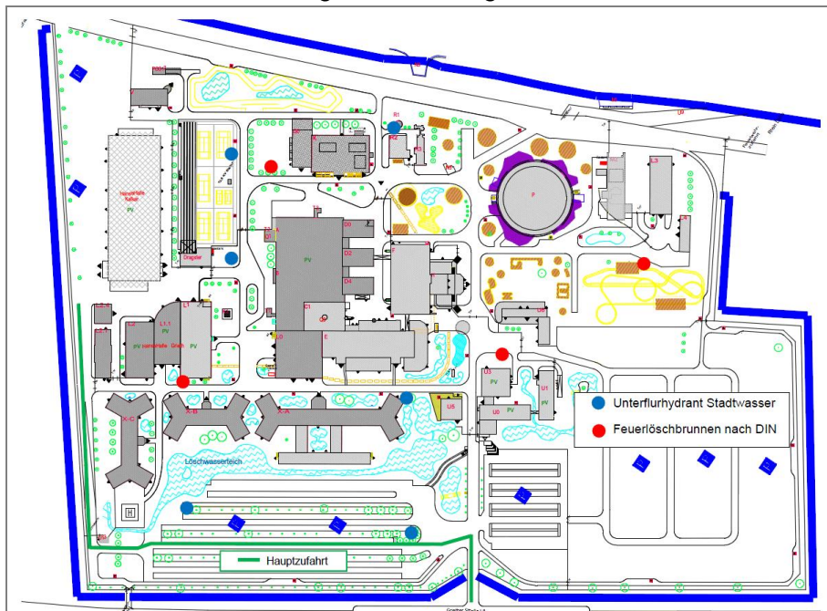
Abbildung 7: Löschwasserversorgung (ohne Maßstab)
