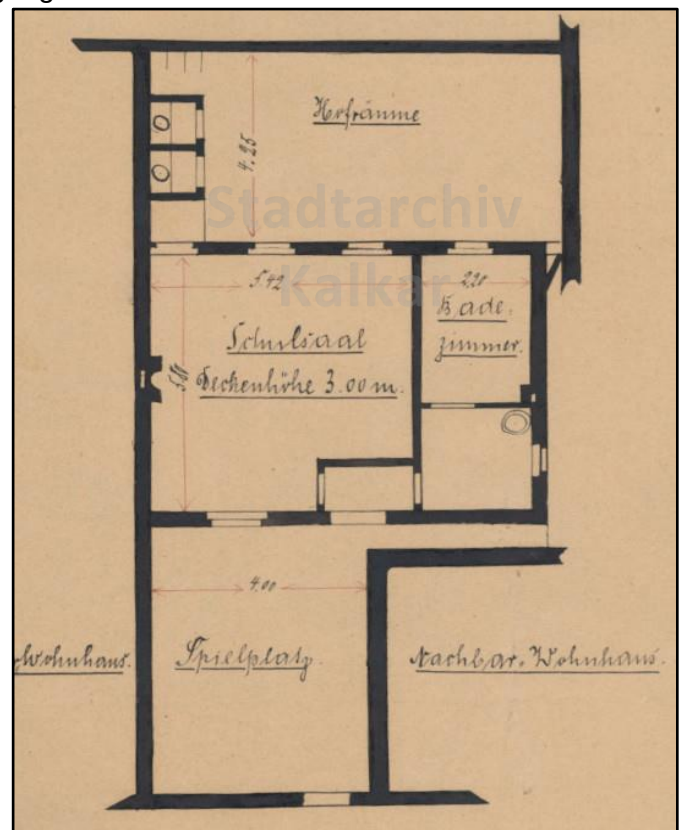
Abb.1: Der von Maurermeister Schweinem im April 1895 angefertigte Grundriss des alten Schulgebäudes.
